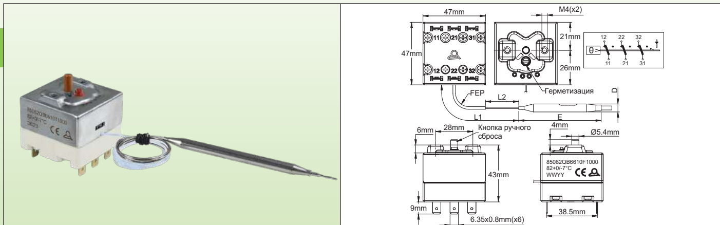
Тип с креплением на 2 винта M4
