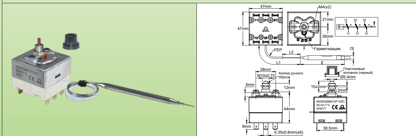
Тип с креплением центральной втулки M10
